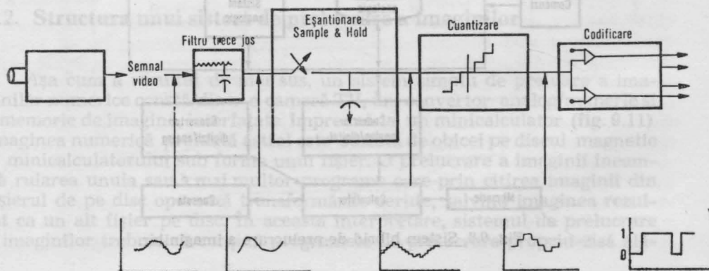
Fig. 9.6. Conversia digitală a semnalelor video.
