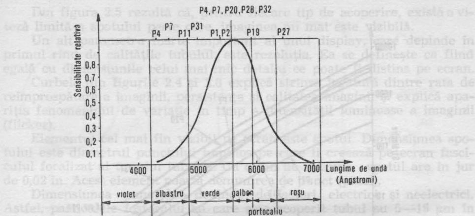
Fig. 2.3. Sensibilitatea spectrală a ochiului pentru diferite tipuri de fosfor.
