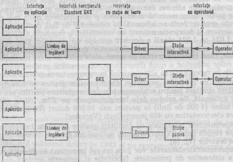
Fig. 1.4. Interfețele GKS.
