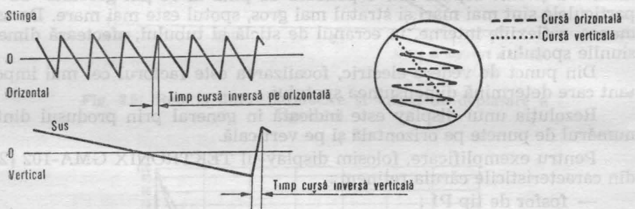
Fig. 2.8. Semnalele de parcurgere raster și imaginea rezultată pe display.
