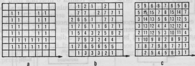
Fig. 9.5. Imaginea 8 \times 8 a literei U : a) binară ; b) cu 3 biți pe pixel și cu zgomote ; c) cu câte 4 biți și variația iluminării pe verticală.
