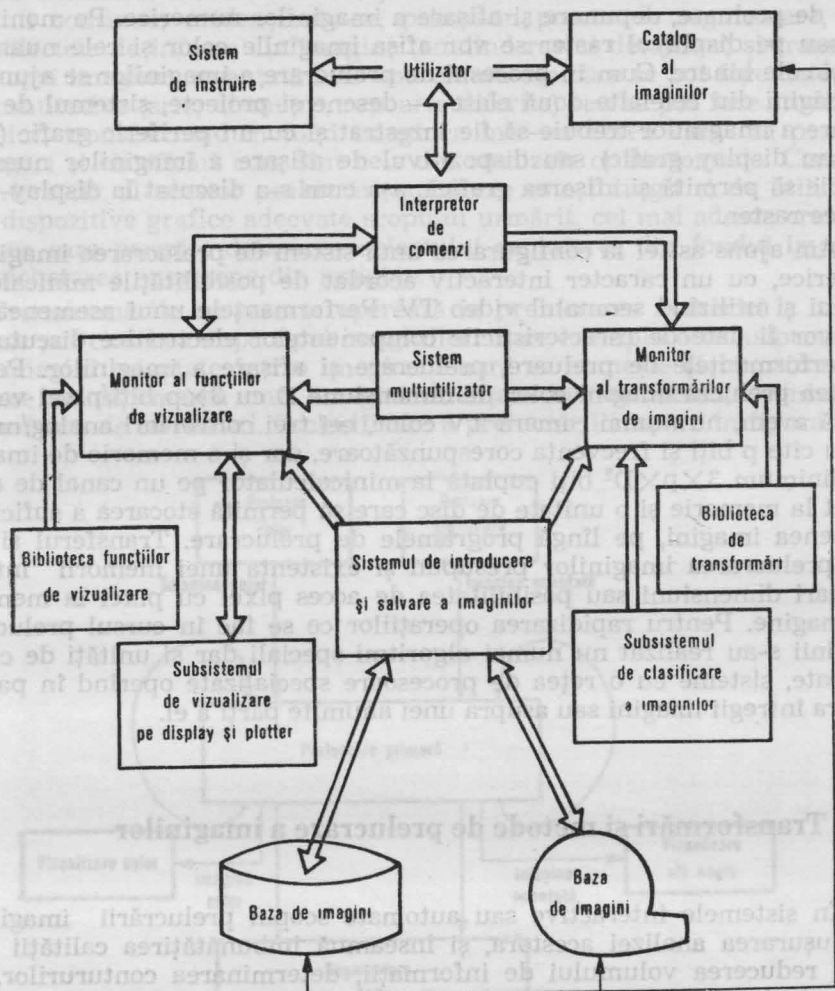
Fig. 9.13. Structura unui sistem de operare specializat pentru prelucrarea imaginilor.
