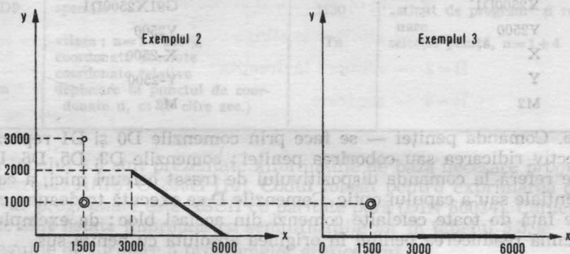
Fig. 3.11. Exemplit de programare a plotterului ARISTO.
