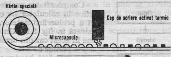
Fig. 3.8. Principiul plotterului termic.
