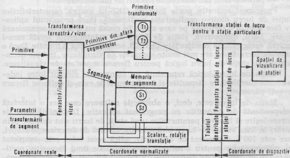
Fig. 5.9. Sisteme de coordonate şi transformări.
