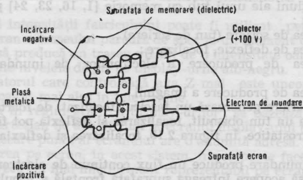
Fig. 2.11. Detaliu asupra zonei suprafeței de memorare.
