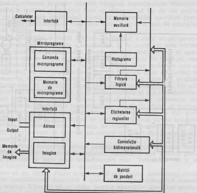
Fig. 9.26. Schema bloc a unui procesor paralel de imagini.
