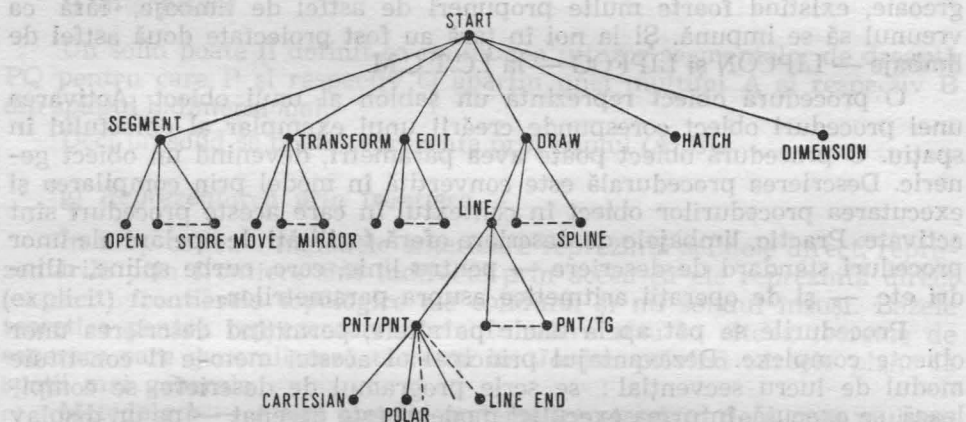
Fig. 6.4. Structura arborescentă a unui meniu de comenzi.
