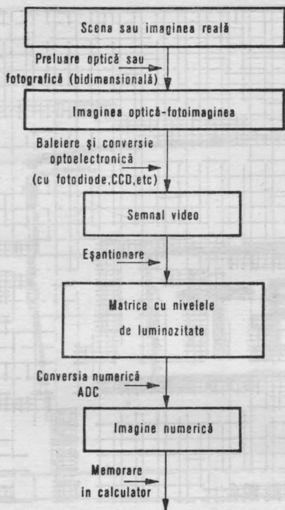
Fig. 9.7. Etapele introducerii imaginii în calculator.
