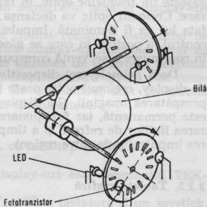
Fig. 2.30. Trackball
