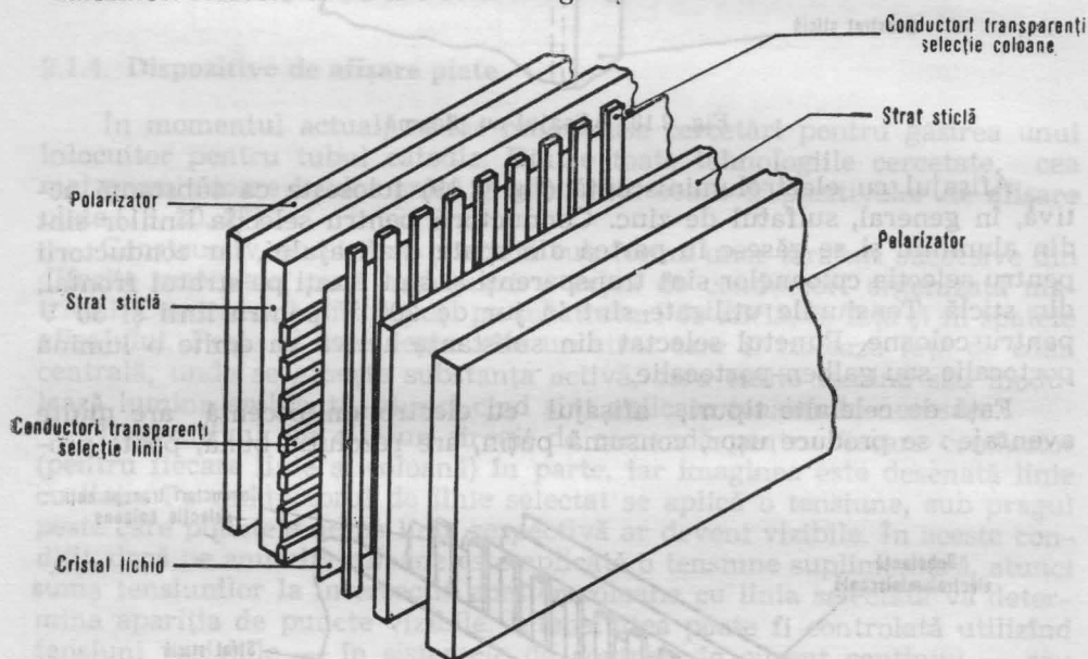
Fig. 2.20. Afișajul cu cristal lichid.
