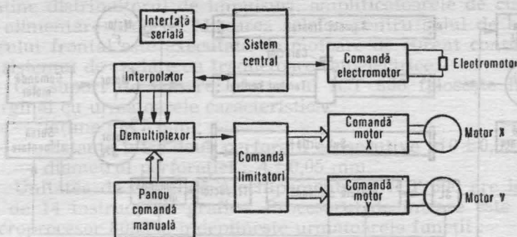
Fig. 4.6. Schema bloc a echipamentului MD 10.
