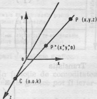
Fig. 5.6. Transformarea perspectivă.
